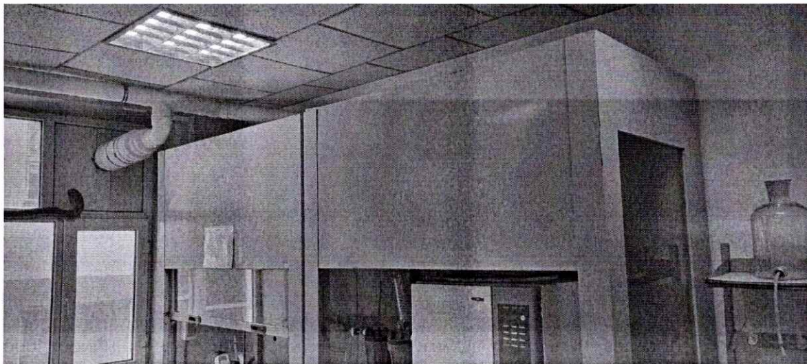
Зураг 2. Агаарын шинжилгээний лабораторид нэмэлт сорох шугам суурилуулсан байдал
