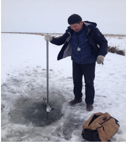
Зургийн тайлбар: Өвлийн улиралд усны өнгөрөлт хэмжиж буй байдал (нэг удаагийн өнгөрөлт хэмжилтэд 3-5 цагийг зарцуулдаг, агаарын температур -15^{\circ}\text{C} -30^{\circ}\text{C} градусуас доош байдаг)
